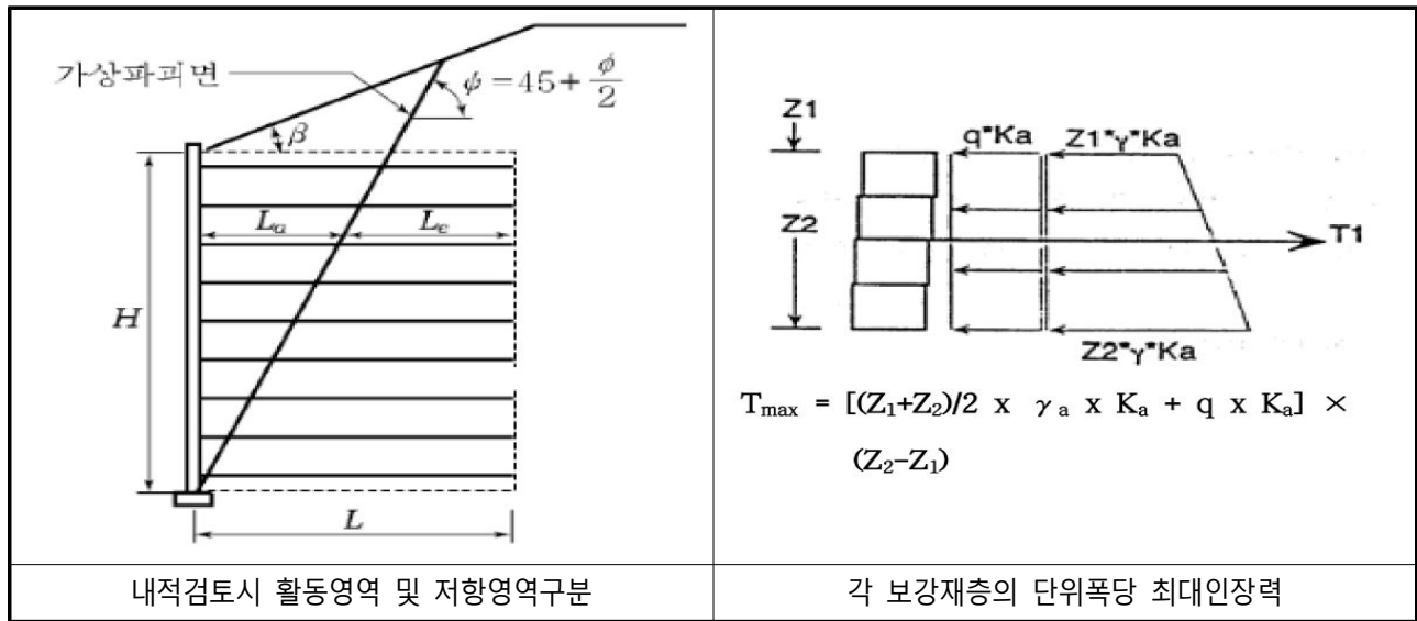
【그림 72.12】 토압작용 모식도
