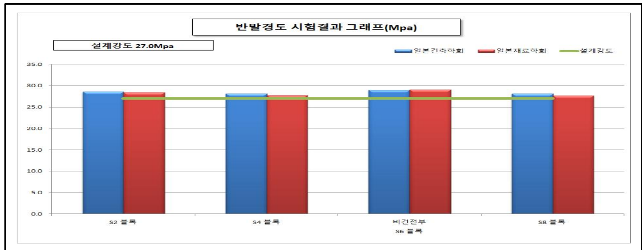
【그림 72.7】 반발경도시험 측정결과
