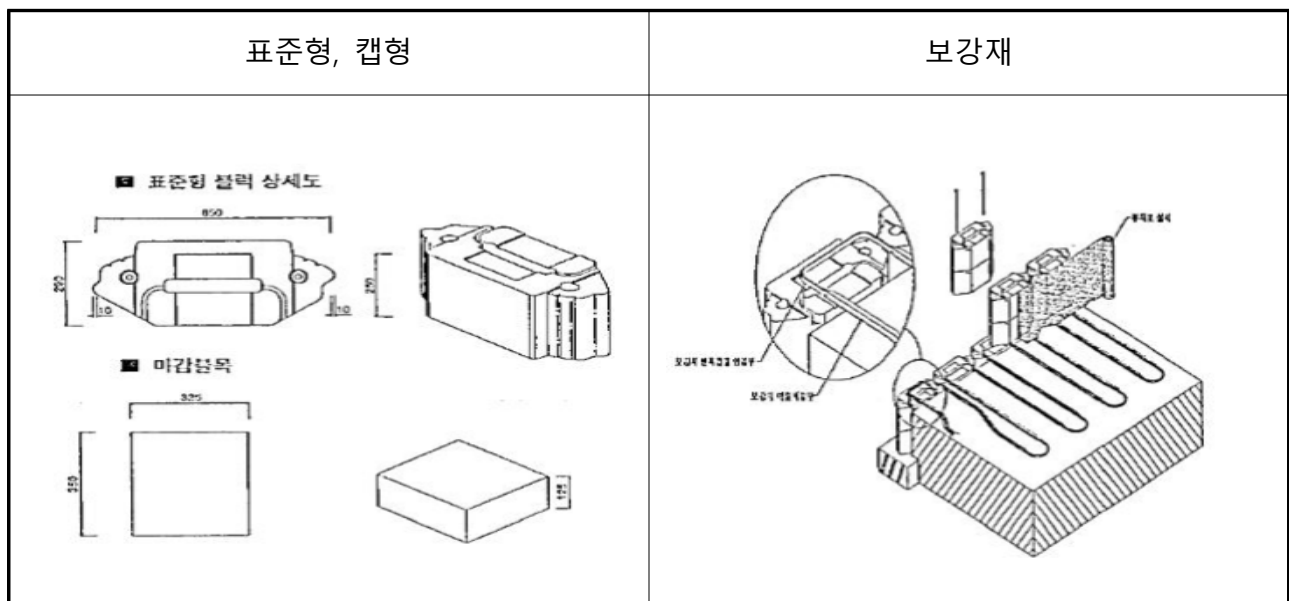
【그림 72.13】 블록 및 보강재 상세도
