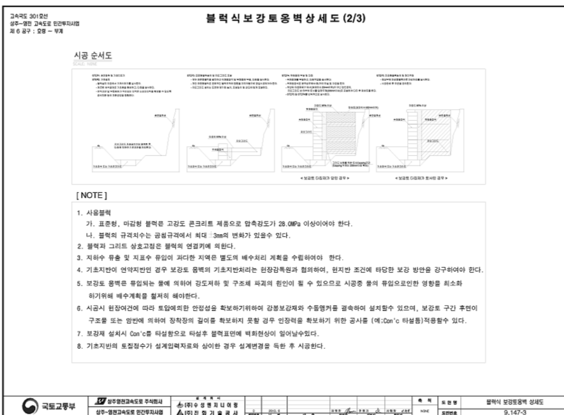
【그림 72.6】 상세도
